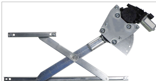
POWER WINDOW RIGHT ALZACRISTALLI ELETTRICO DX
