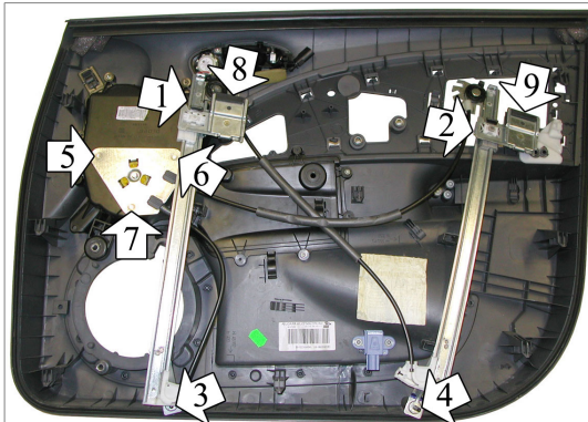
A POWER WINDOW LEFT ALZACRISTALLI ELETTRICO SX
